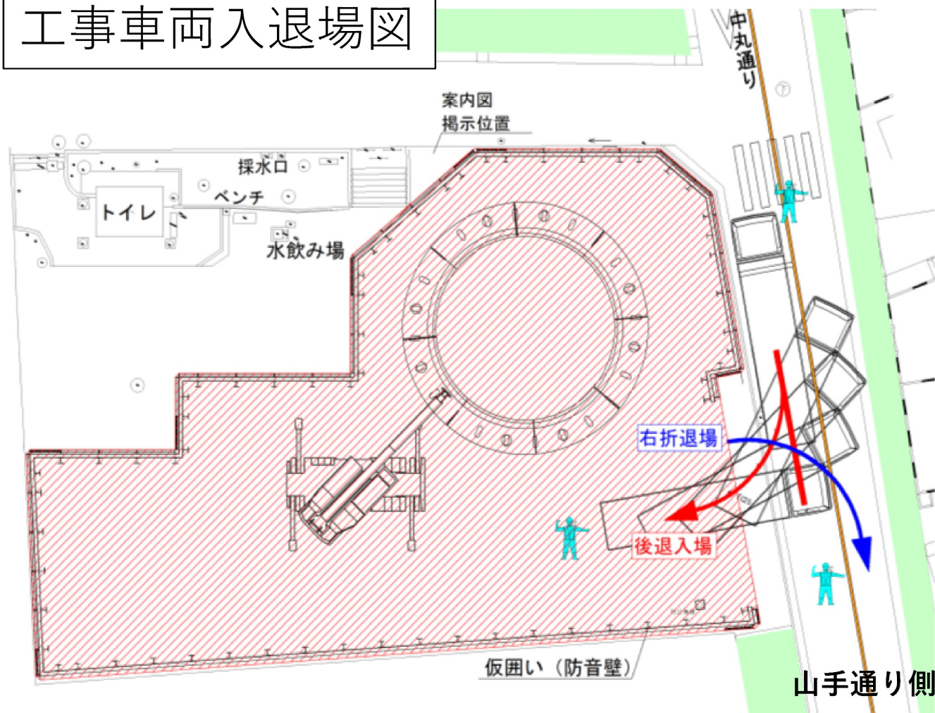
10 t ミキサー車
